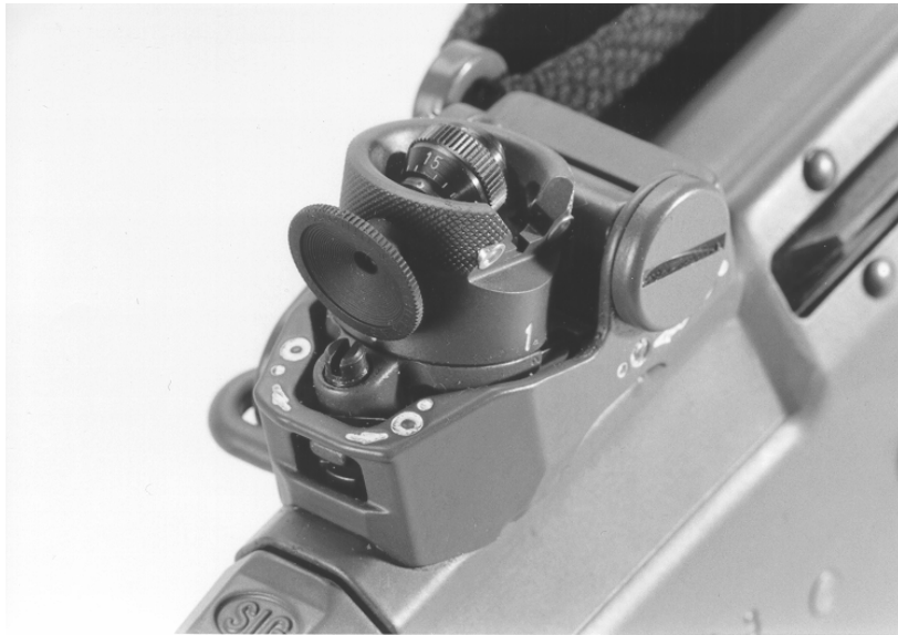
Bild 1: Irisblende zu Sturmgewehr 90 Modell Grünig + Elmiger
